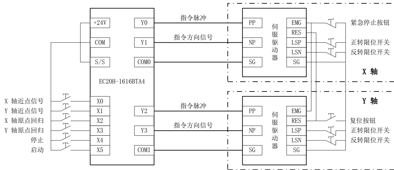
设备接线示意图
