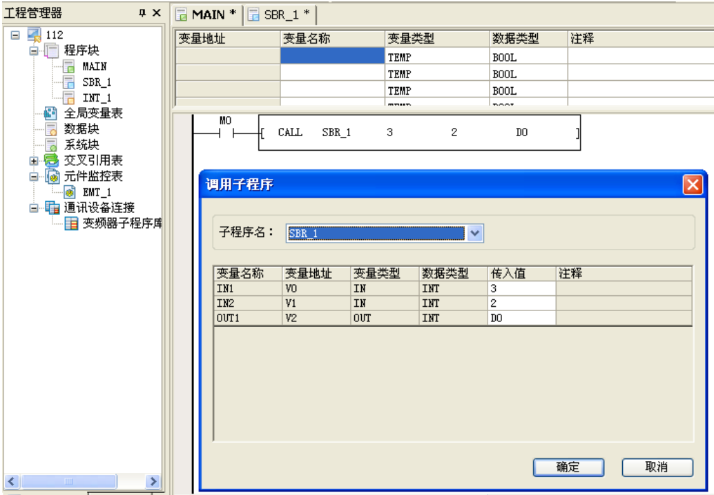
图4-12 调用子程序
