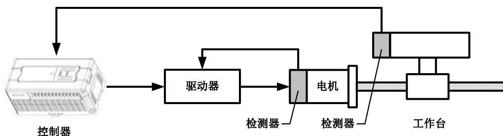
图11-4 闭环控制系统简图
