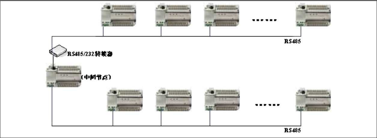
图10-8 N:N 多层网络
