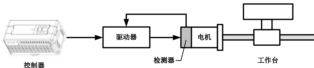
图11-5 半闭环控制系统简图
