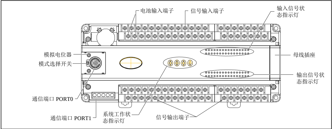
图1-2 PAC2L 系列主模块的外形结构与部件布局
