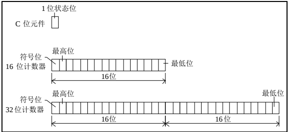
图3-4 C 元件
