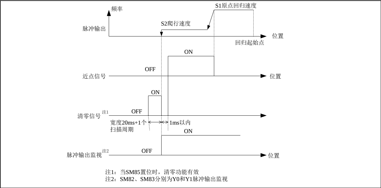
时序图
