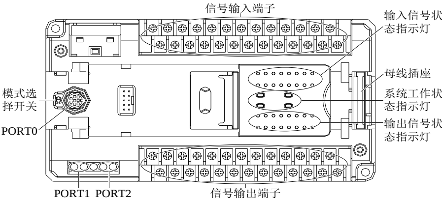
图1-3 PAC2H 系列主模块的外形结构与部件布局
