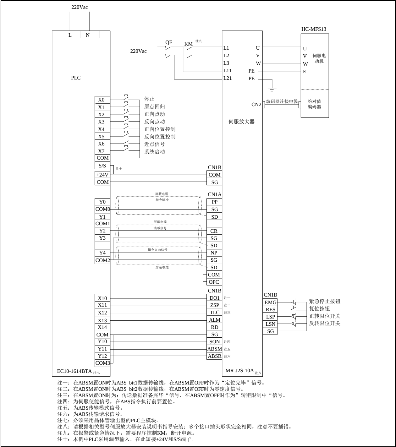
图11-8 设备接线示意图
