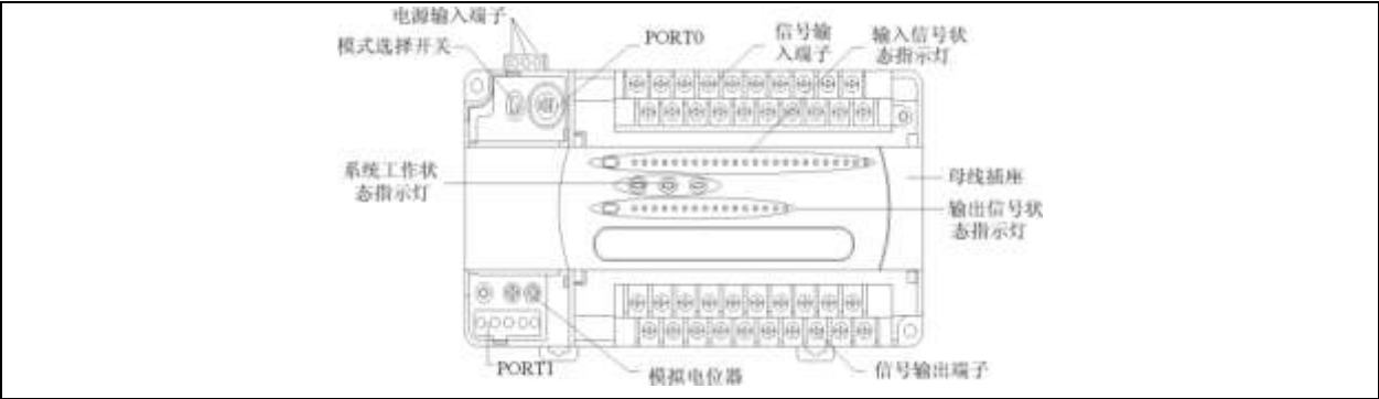
图1-1 PAC1 系列主模块外形结构
