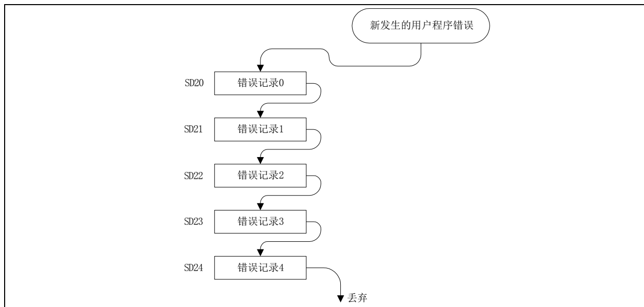
图2-19 错误编码的压栈操作过程
