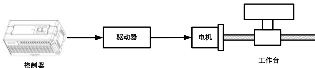
图11-3 开环控制系统简图
