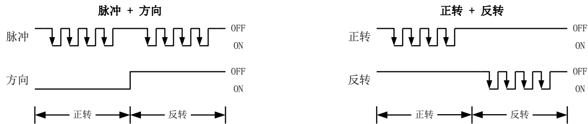
图11-7 脉冲输出形式的定义
